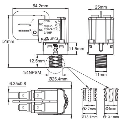
Filetage 1/4" NPSM
